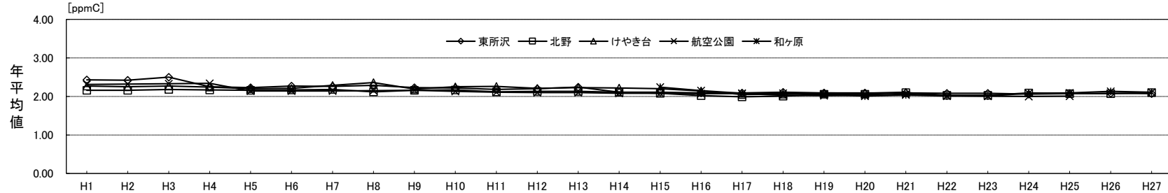
全炭化水素(THC)の経年変化
